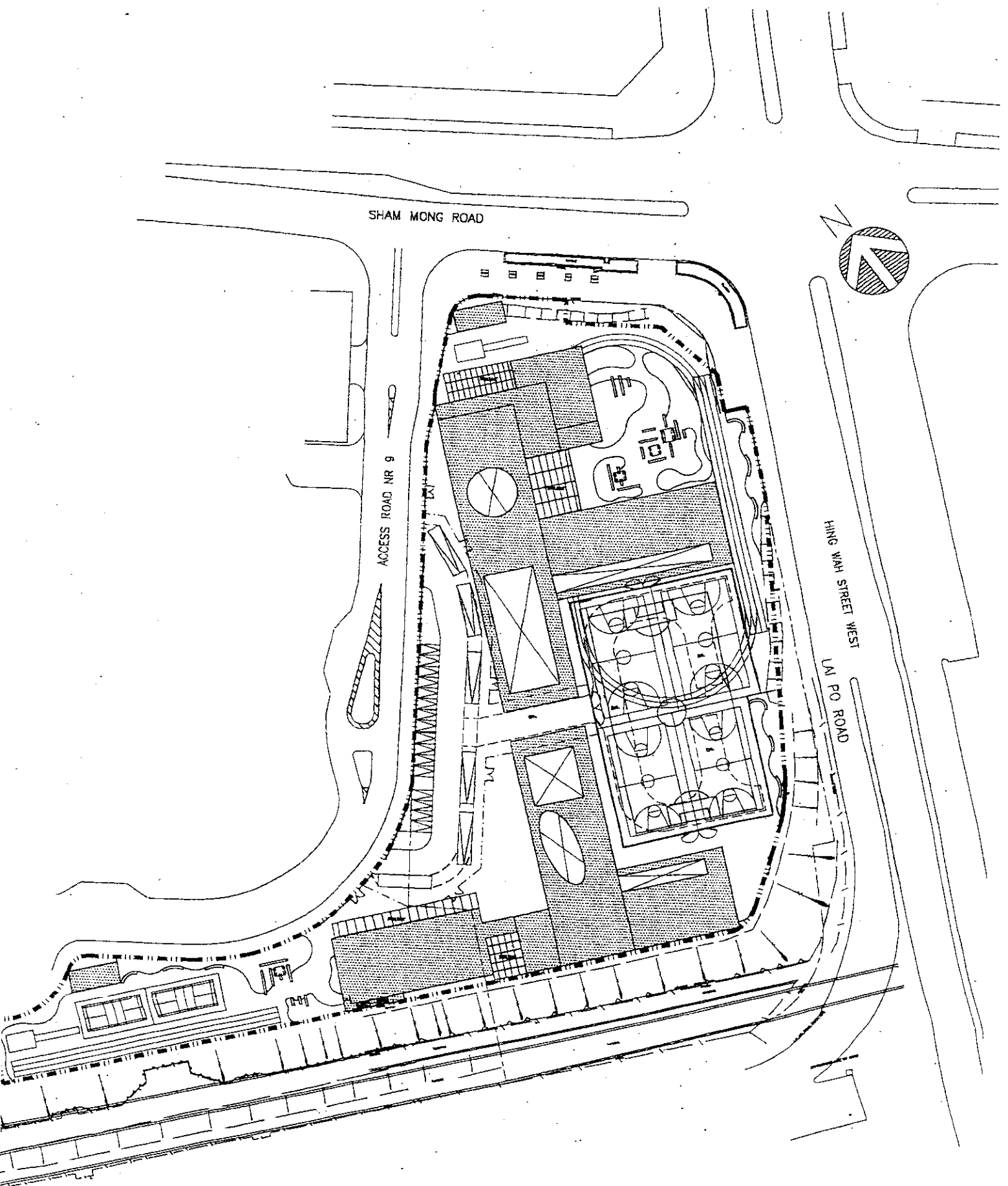
圖一：西九龍填海區第十號地盆一所小學(3319EP)及一所中學(3256ES)的校舍設計平面圖
