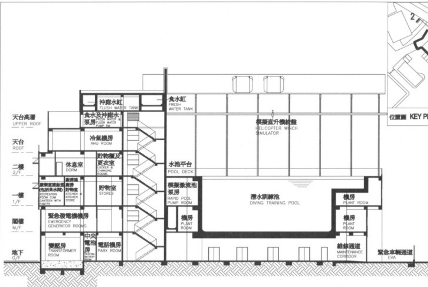
切面圖二 SECTIONAL PLAN 2
