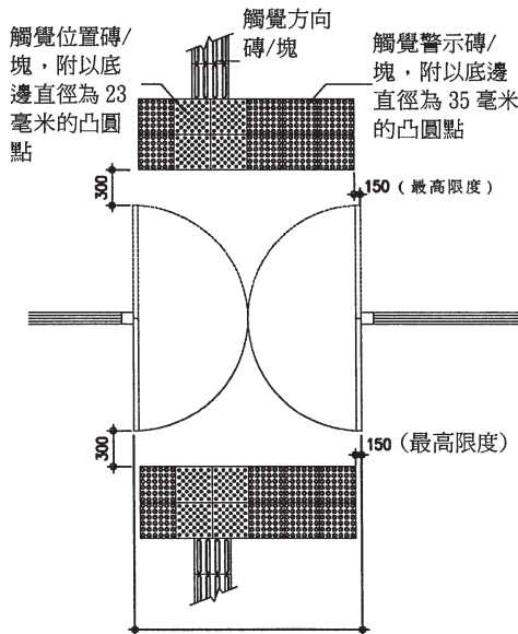
(b) 雙向掩門入口的觸覺警示帶
