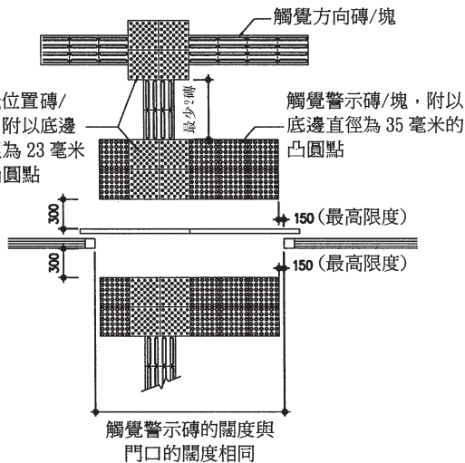
(b) 雙向掩門入口的觸覺警示帶
