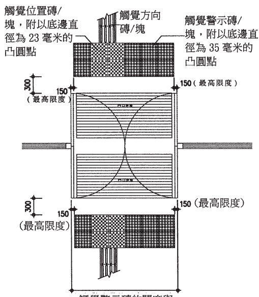
(c) 位於入口設有門口地毯的觸覺警示帶
