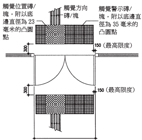
(a) 單向掩門入口的觸覺警示帶
