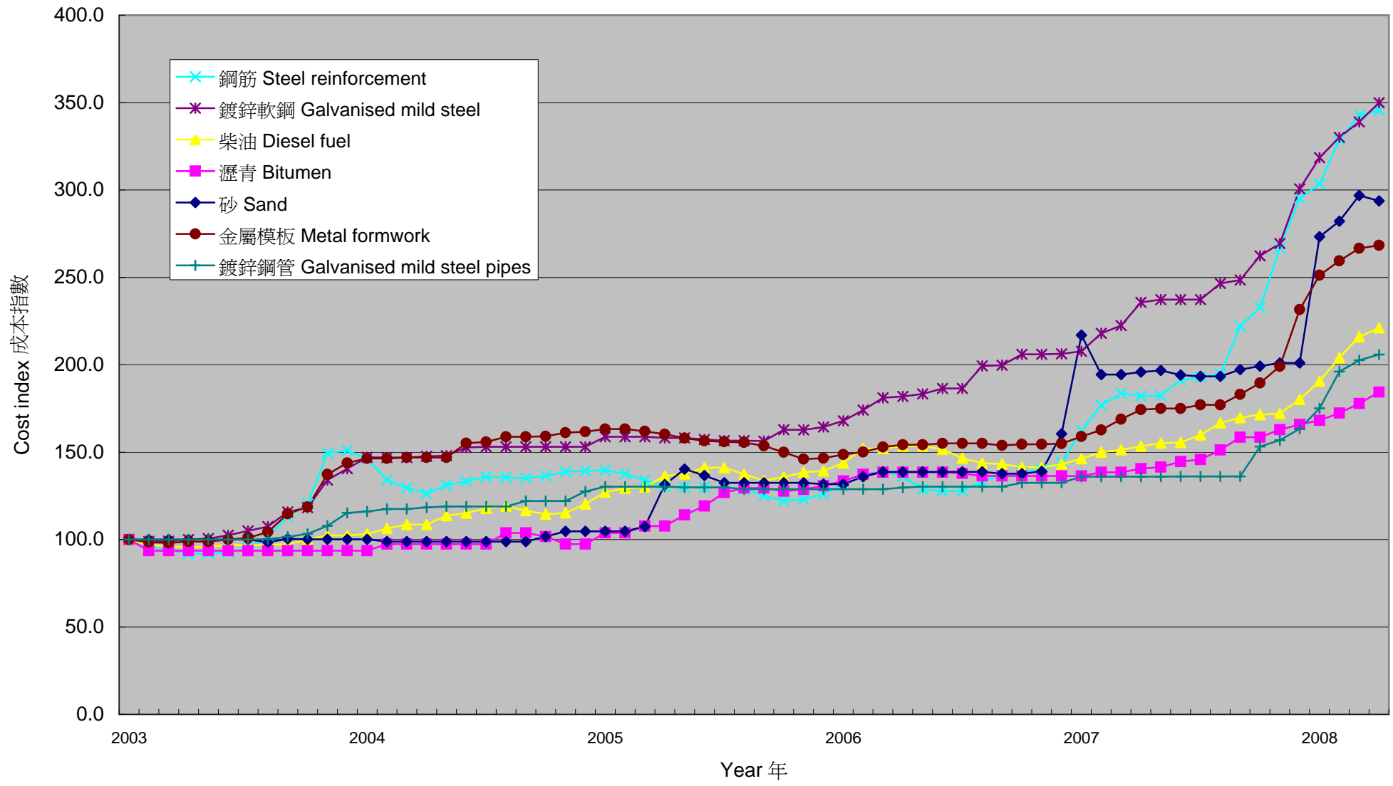
公營建築工程的材料成本指數 (2003年4月=100) (2003年4月至2008年7月) Index Numbers of Costs of Materials used in Public Sector Construction Projects (April 2003=100) (April 2003 – Jul 2008)
