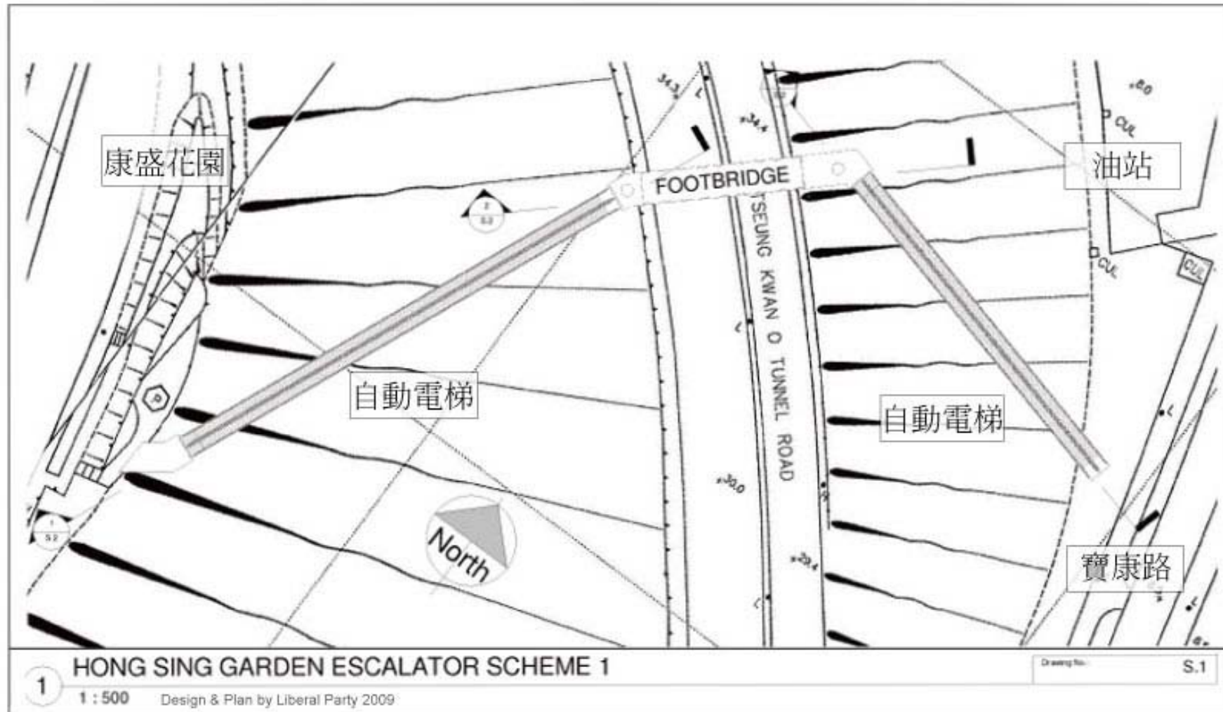
康盛花園與寶康路之間興建自動電梯系統建議圖則
