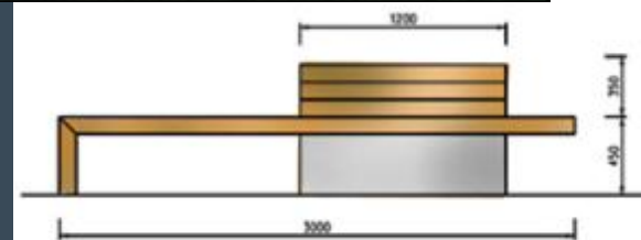
Elevation 立面圖
