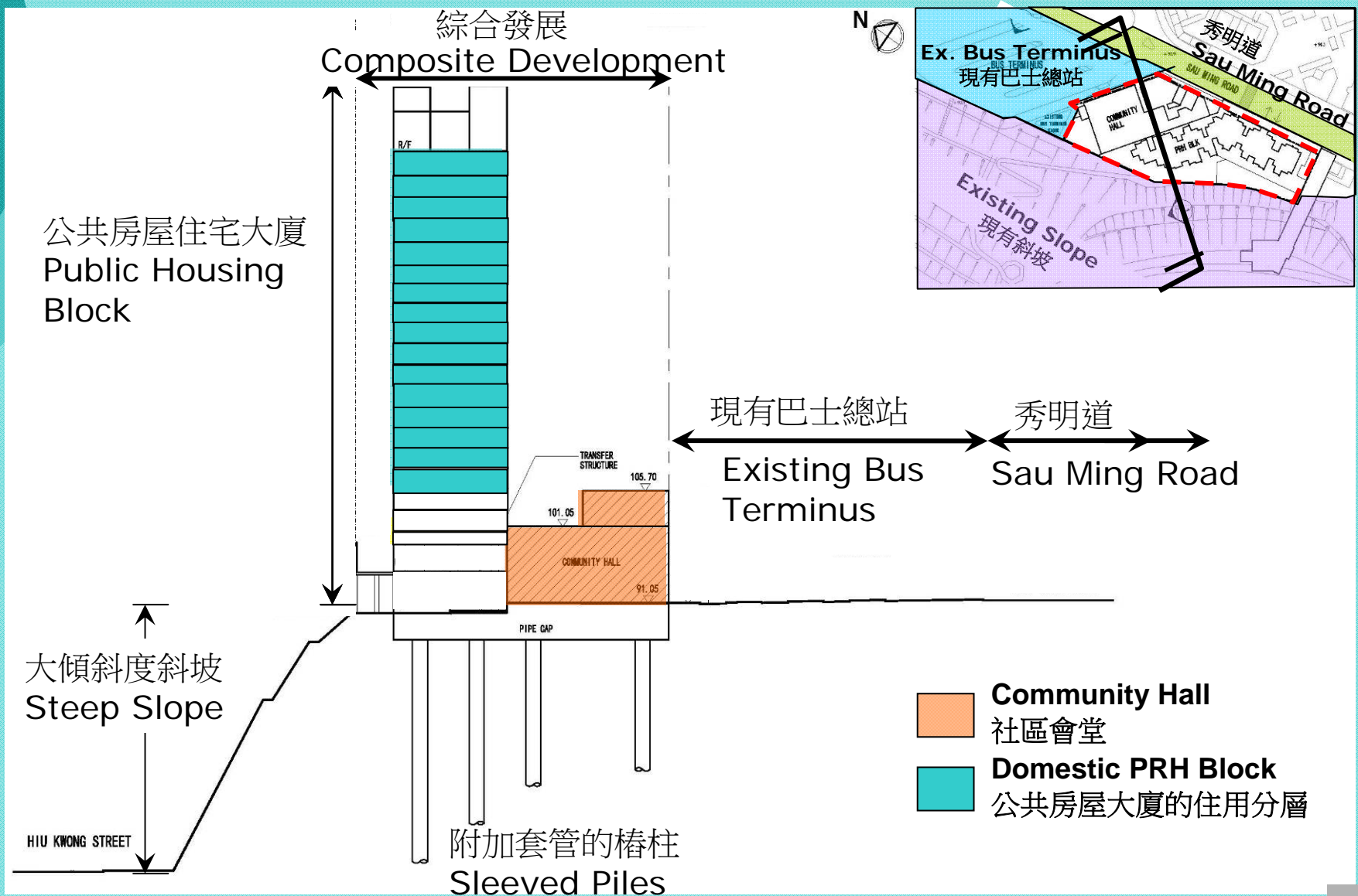
MAIN SITE SECTION 地盤主要切面圖
