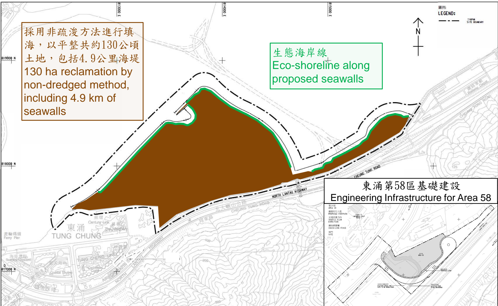
工程項目平面圖 - 東涌新市鎮擴展 - 填海及前期工程 PROJECT LAYOUT PLAN - TUNG CHUNG NEW TOWN EXTENSION - RECLAMATION AND ADVANCED WORKS
