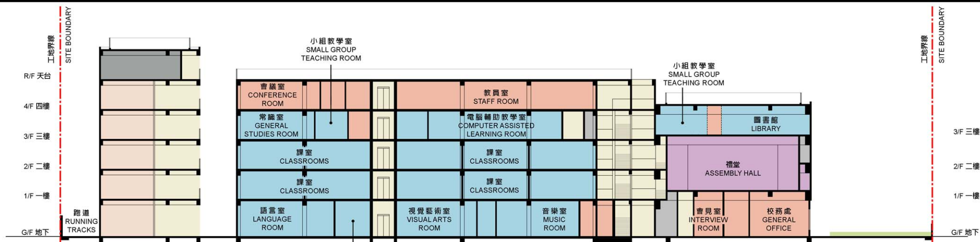
剖面圖 A-A SECTION A-A
