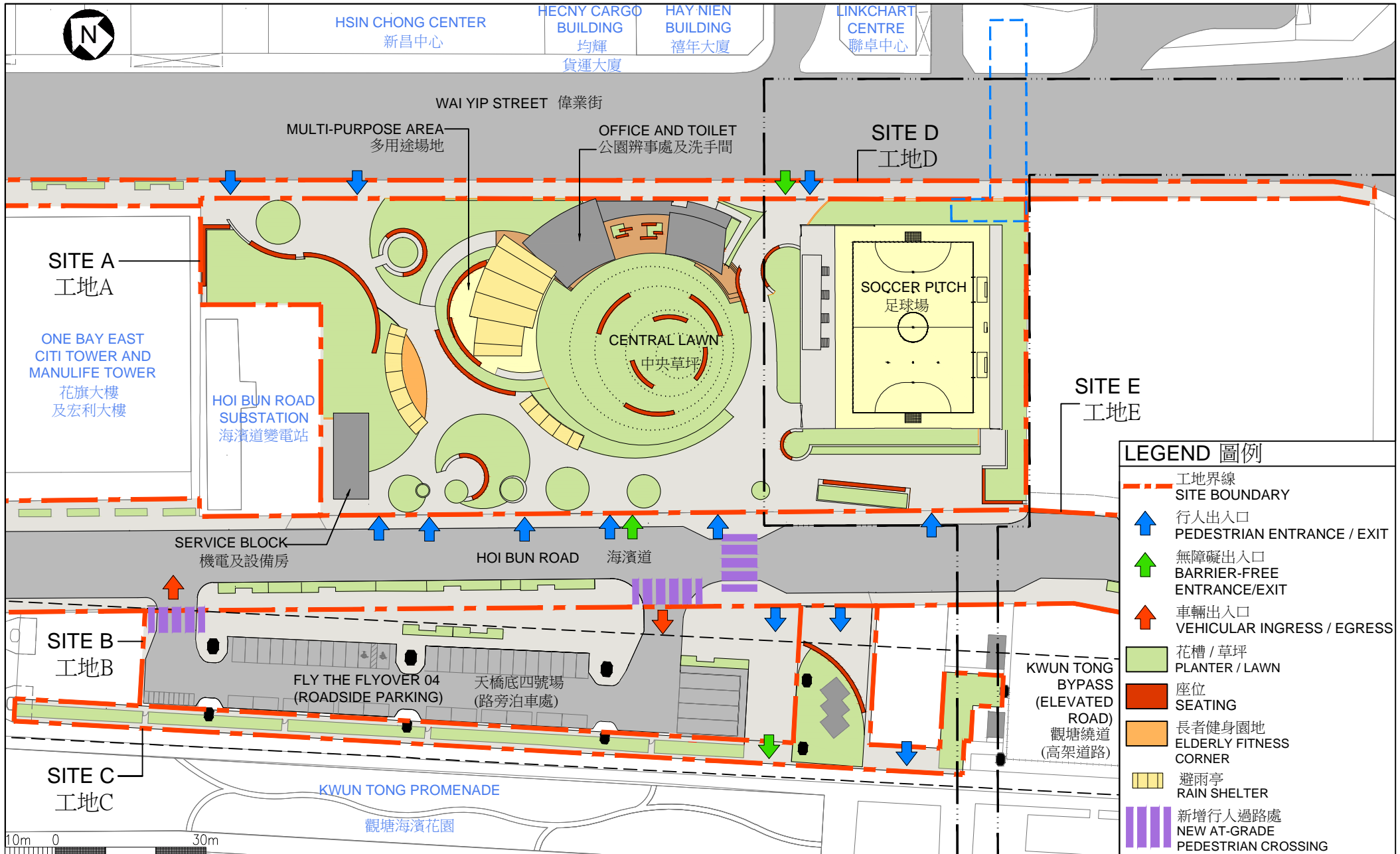
工地平面圖 (局部) SITE PLAN (PARTIAL)
