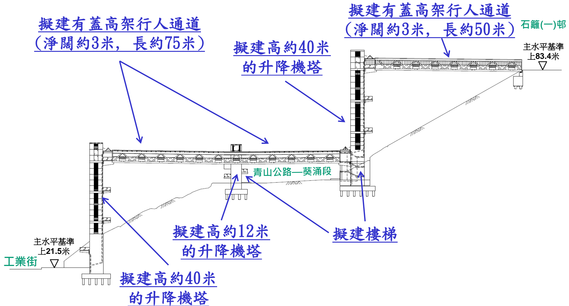
立面圖
