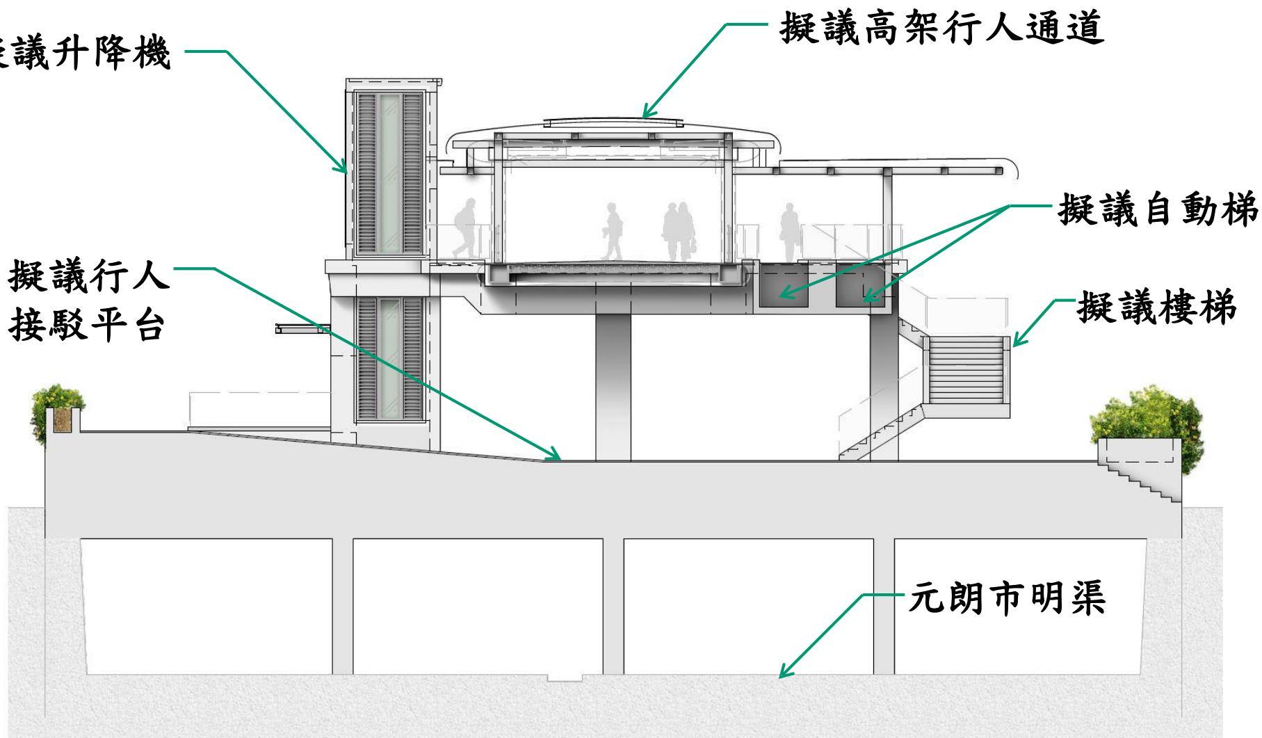
切面 I - I
