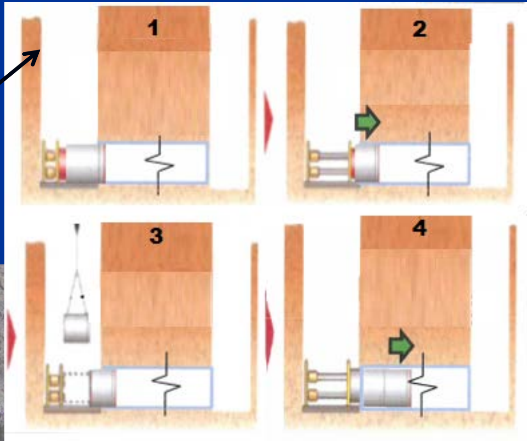
內套喉管修復示意圖
