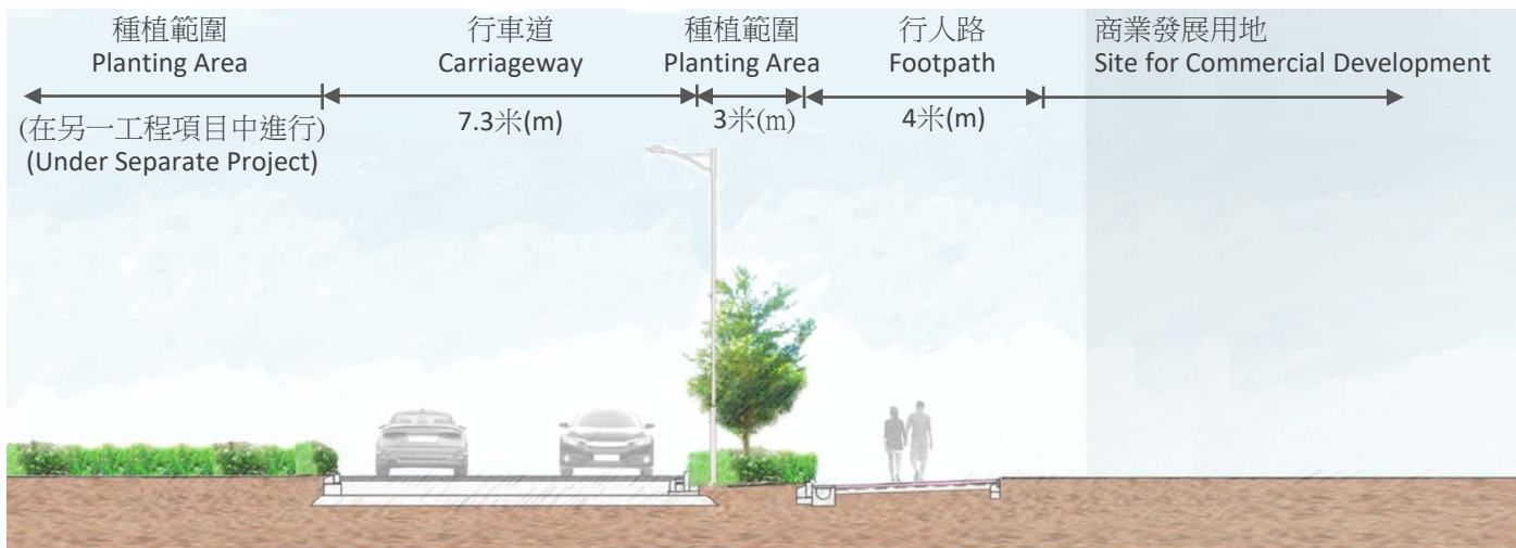
擬議L10路(北段) (構想圖) 橫切圖 A - A
