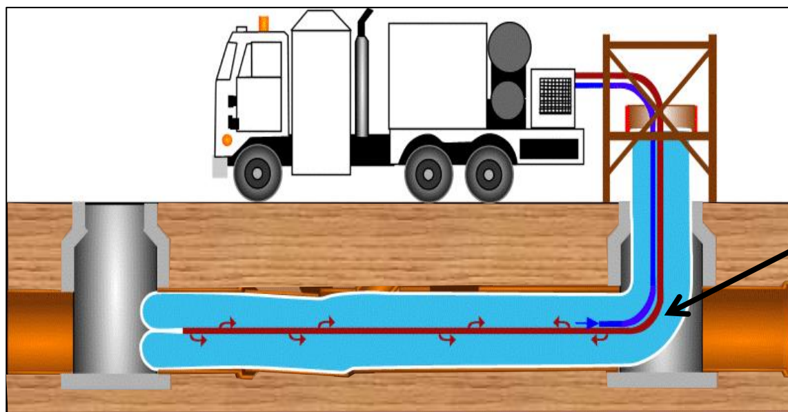
(1) 原位固化內襯修復示意圖
