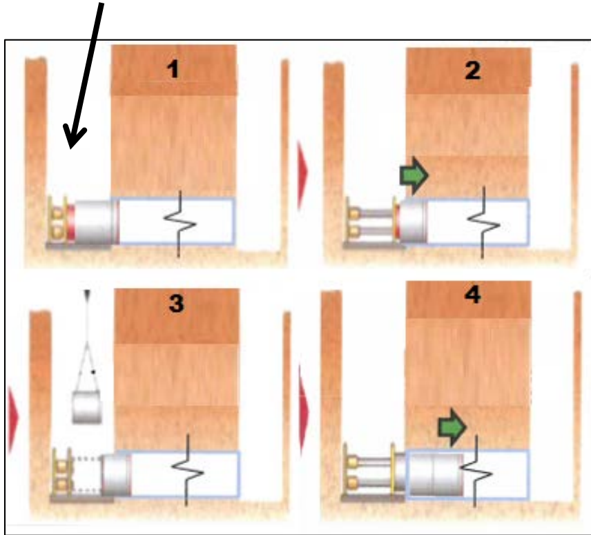
(2) 內套喉管修復示意圖
