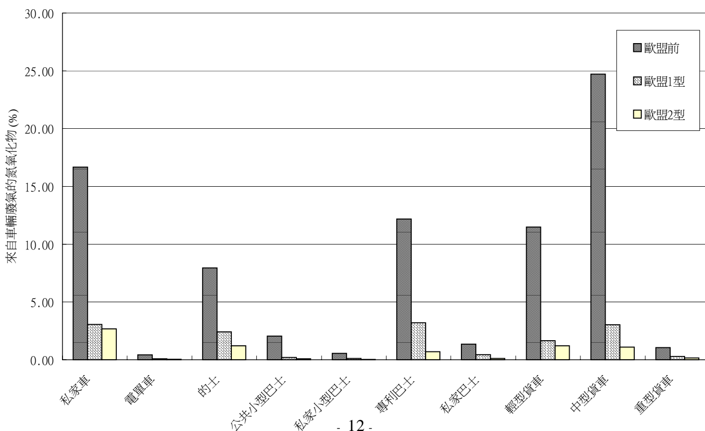
氮氧化物
