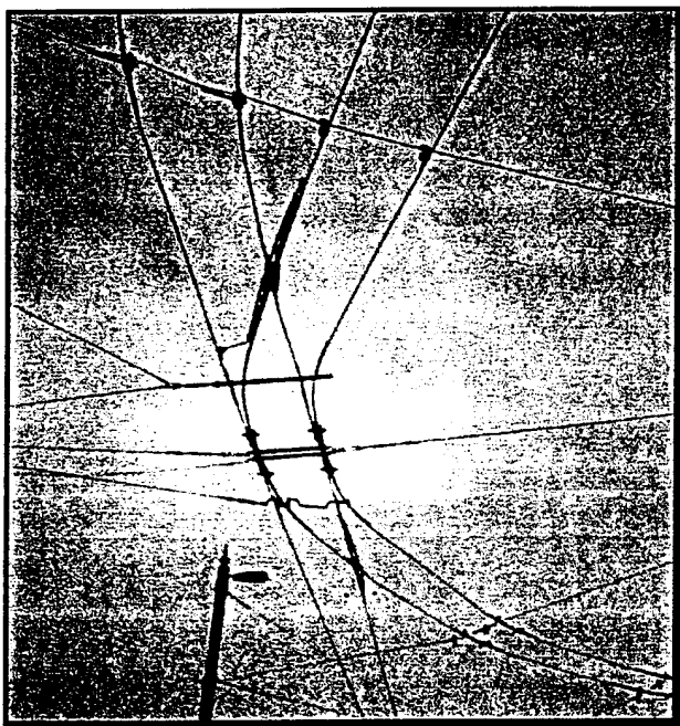
圖五 一系列用於英國的現代架空電纜設備。前方（圖頂）為剛性懸掛設備而後方為彈性懸掛設備，中間為對向「轍叉」。 (Peter Price)
