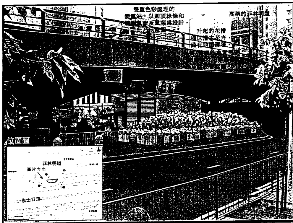
圖六 這圖展示位於菲林明道天橋底的牽引性變電站外貌。 (背景照片：Townland Consultants Limited)
