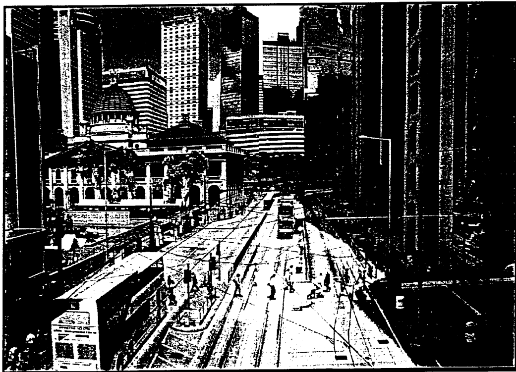
圖七 這圖展示在德輔道中的架空電纜及牽引柱，此由太子大廈行人天橋望向立法會大樓。 (背景照片：Barnaby P. Smith)
