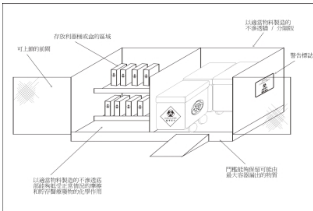
圖3：醫院和大型診所的醫療廢物貯存設施簡圖
