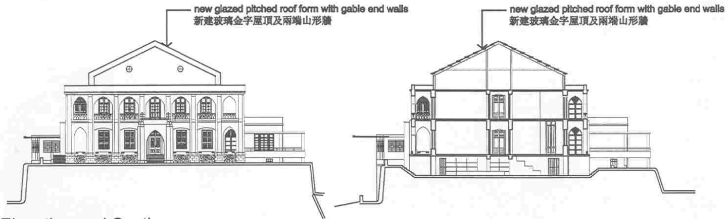
Elevation and Sections 立面圖及剖面圖 1:400
