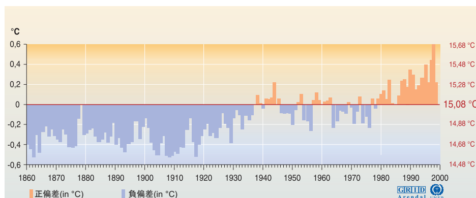
圖1：地球平均表面溫度的上升趨勢
