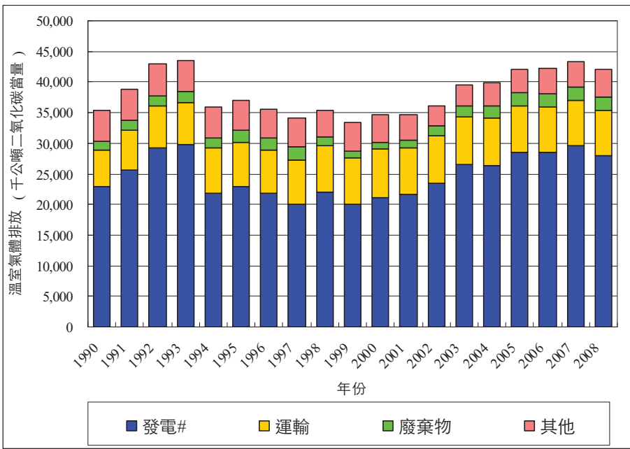
圖4：1990年至2008年香港溫室氣體排放趨勢
