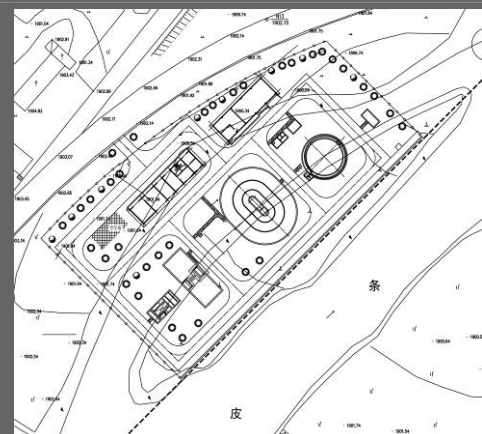
臥龍污水廠 總平面圖
