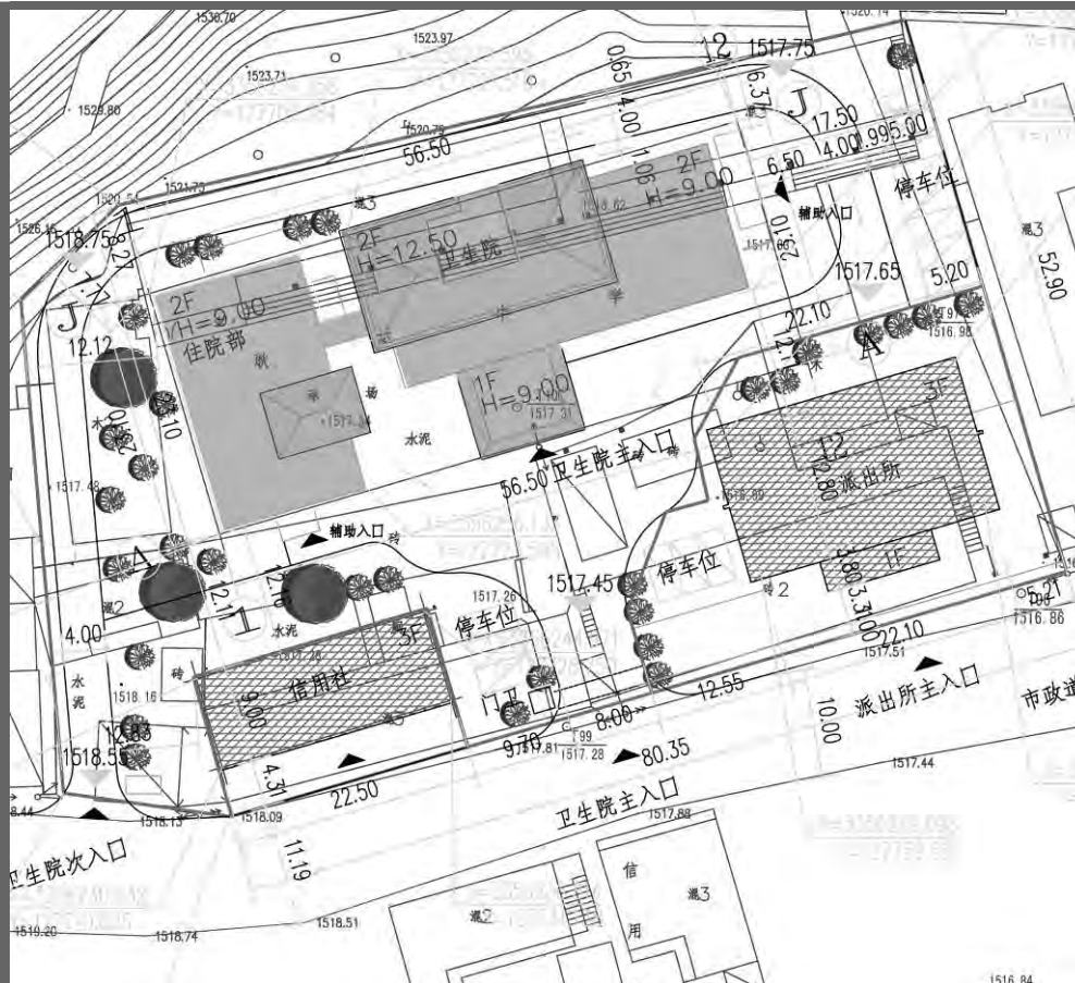
耿達衛生院 總平面圖
