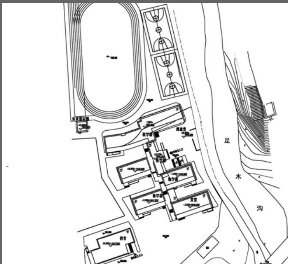
總平面圖
