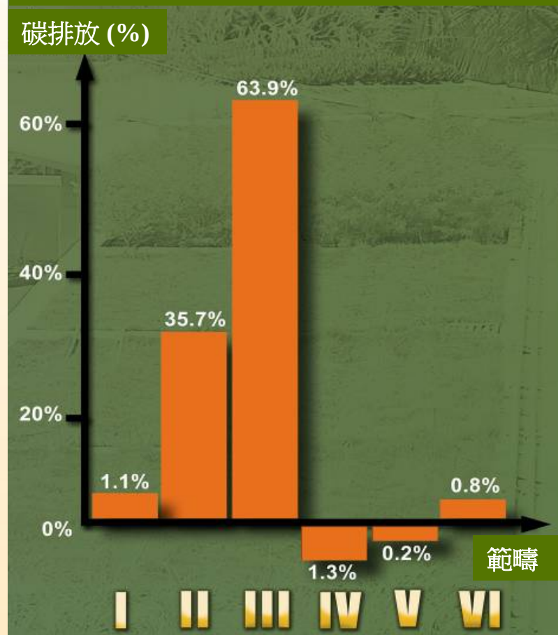
碳排放量估算六個範疇的比較 (啟德 1A區)
