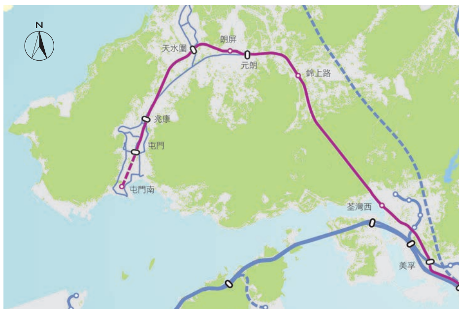
圖6.5：屯門南延線的初步構思
