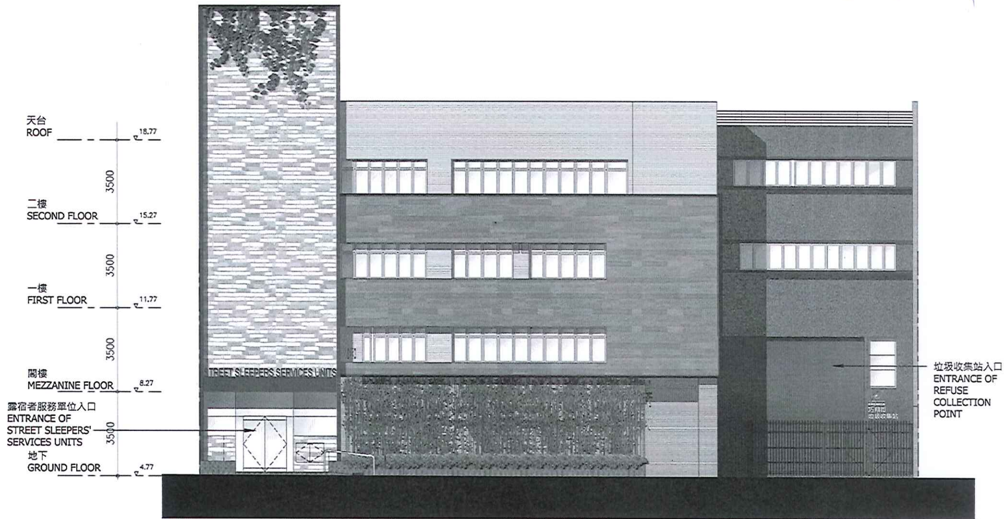
西面立面圖 WEST ELEVATION
