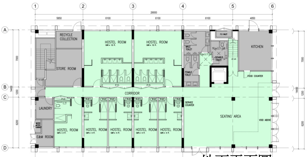
地下平面圖
