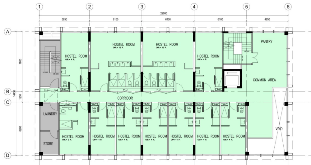
一樓平面圖
