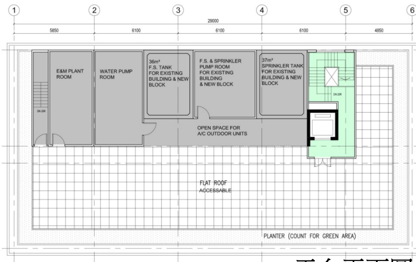
天台平面圖
