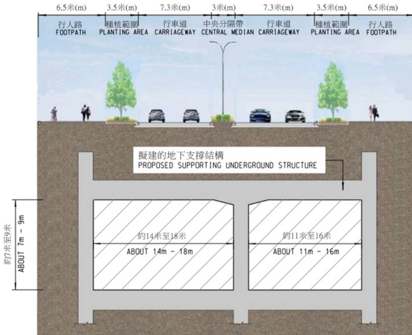
橫切面 B-B Section B-B
