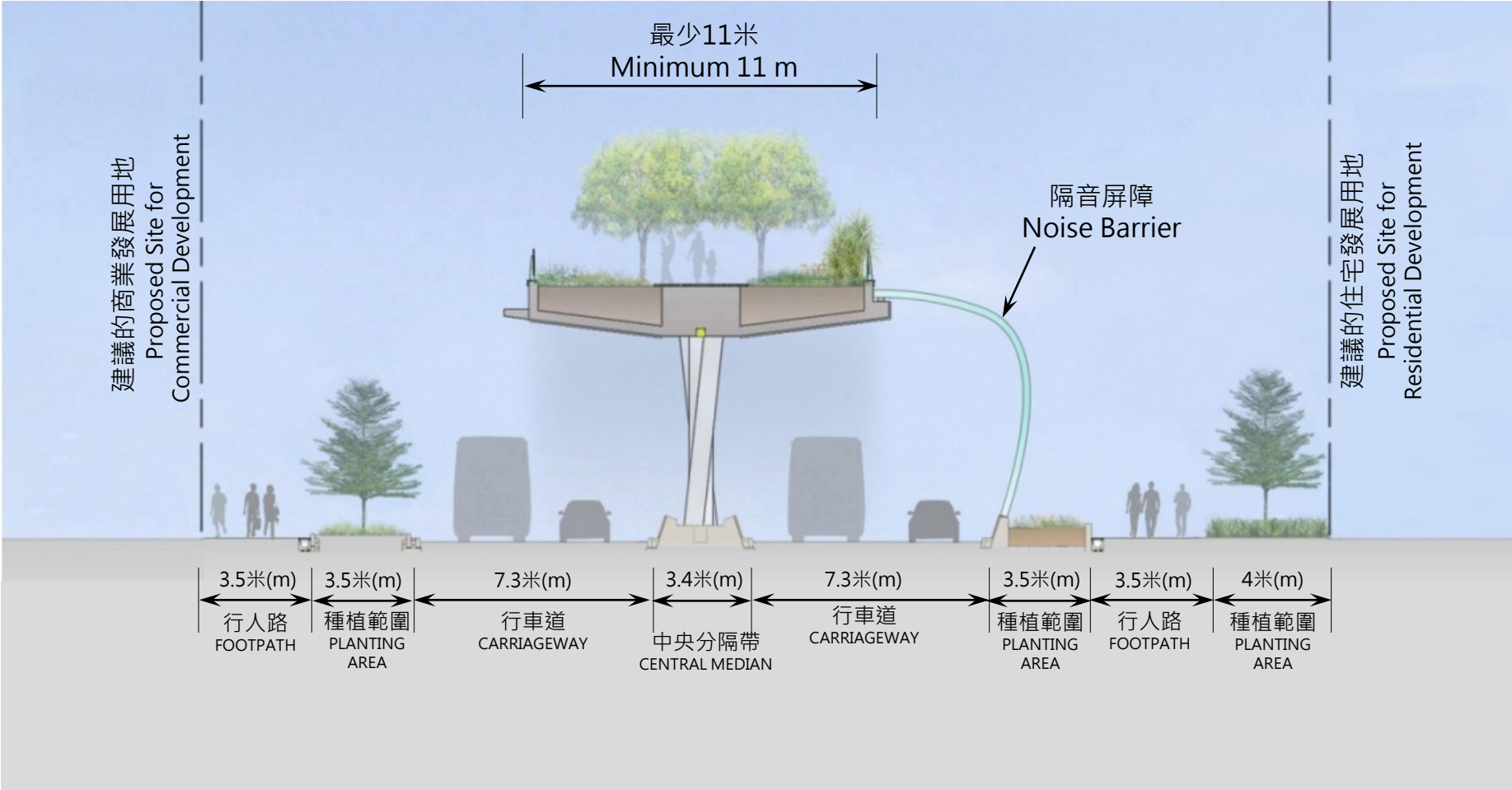
橫切面 A-A Section A-A
