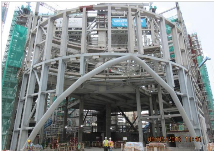
Primary Steel Frame (Entrance) 主要鋼結構 (入口)
