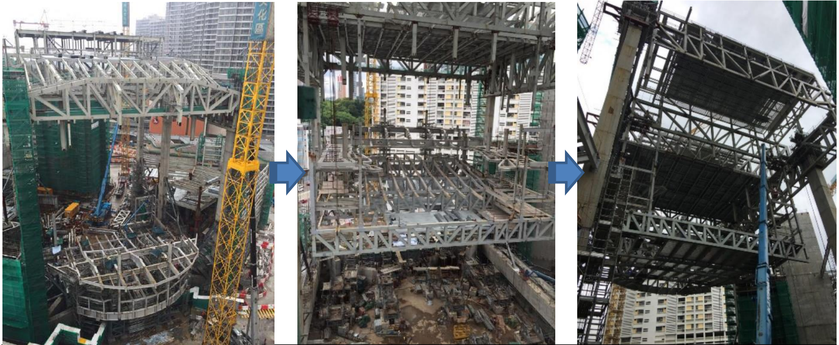
May 2016: Erection of the Theatre Steel Structure (The main theatre structure weighs 2 400 tonnes) 2016年5月：劇院主要鋼結構支架整體吊裝 (主劇院結構支架重約 2 400 公噸)
