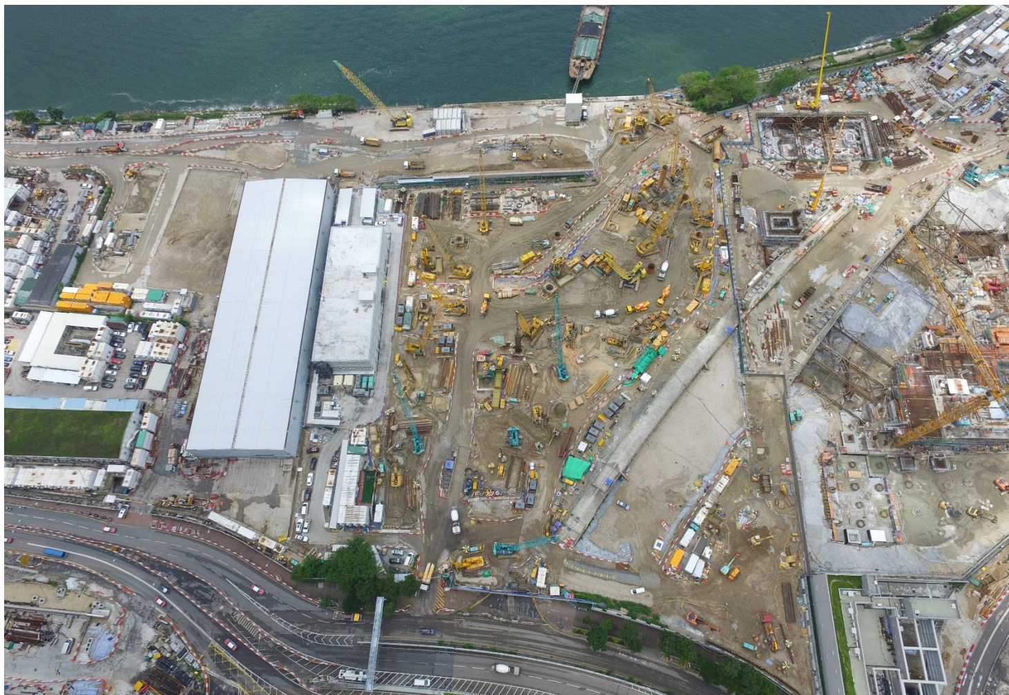
Foundation works in progress 地基工程進行中
