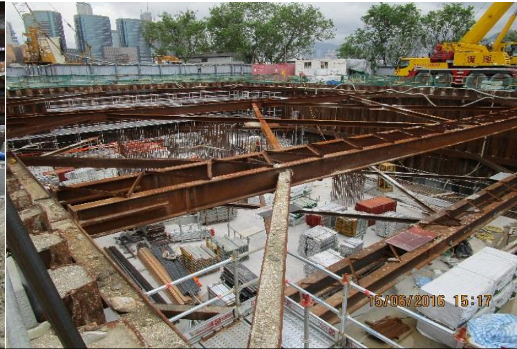
B2 Slab & Sump Pit Construction at District Cooling System 在區域供冷系統區建造第二層地庫樓板及集水坑
