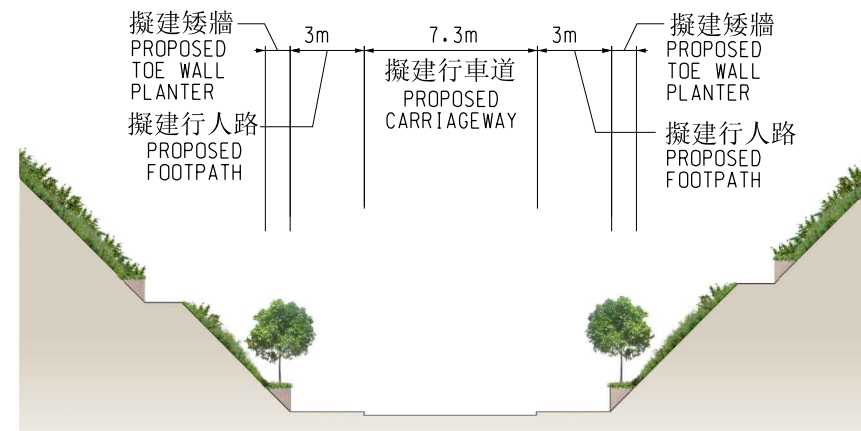
剖面圖 B - B SECTION B - B
