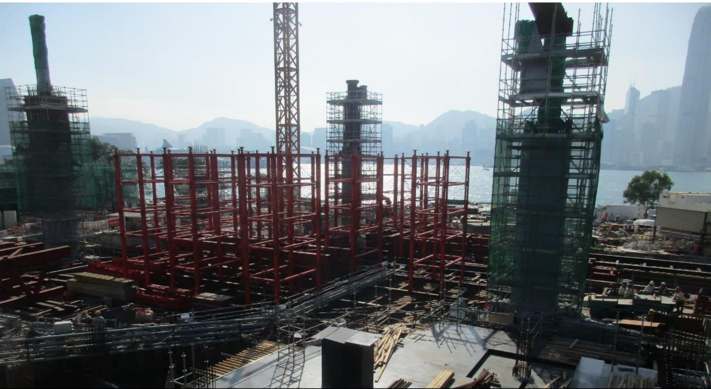
Temporary Works for Trusses 3 and 4 第三及四號桁架的臨時工程
