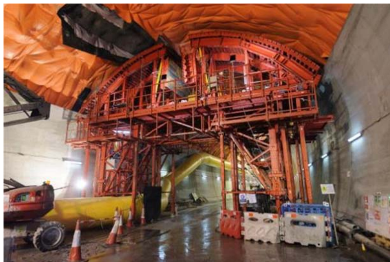
越位隧道正進行結構工程
