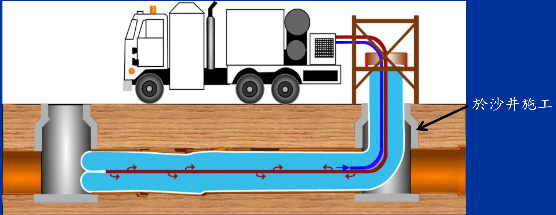
原位固化內襯修復示意圖
