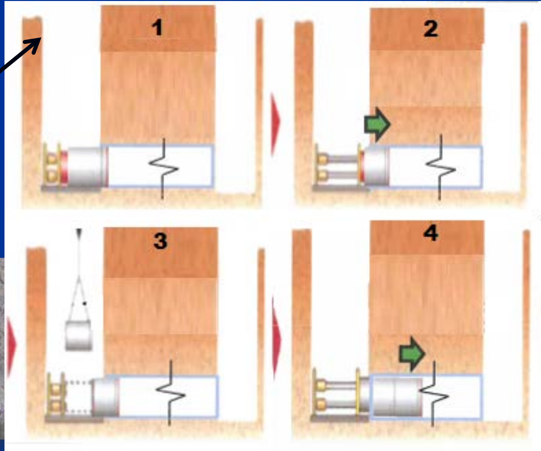
內套喉管修復示意圖
