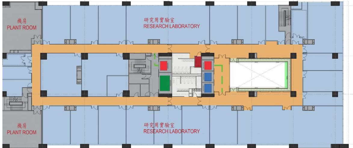
五至七樓平面圖
