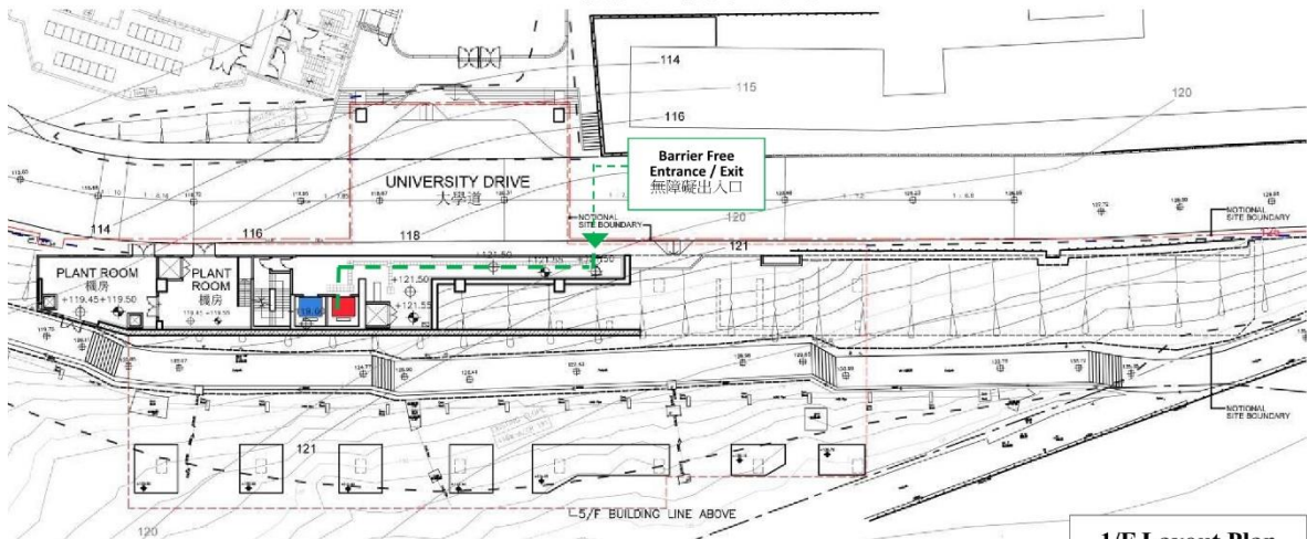
1/F Layout Plan 一樓平面圖
