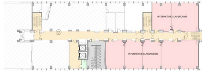
三樓平面圖 Second Floor Plan
